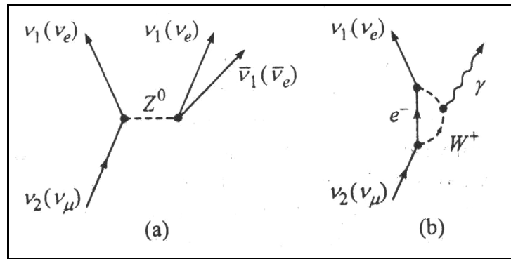
Рис. 18. (а) Распад нейтрино на три нейтрино и (б) радиационный распад \nu_2 \rightarrow \nu_1 + \gamma . Имеются другие экзотические каналы распада, например с испусканием майорона (по работе 103 )
