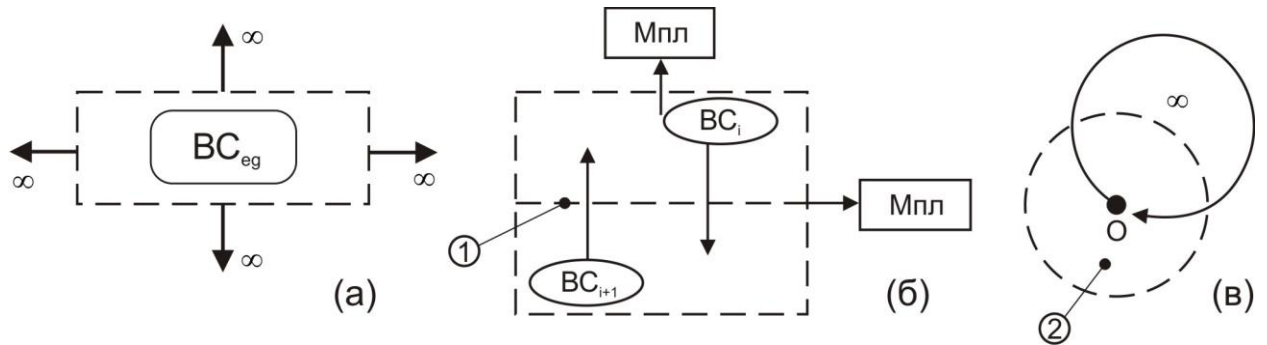
Рис. 15. Исходный фон для формирования вселенной в вариантах (а), (б) и (в): BC_{ед} – предположение одной вселенной в Мироздании – нашей Вселенной; M_{пл} – бесконечная мультипликация; BC_i и BC_{i+1} – соседние вселенные в их множественности; 1 – циклически изгибающаяся «мембрана»: если BC_i расширяется, то BC_{i+1} сжимается до точечной сингулярности в момент, когда BC_i занимает предельный объем; 2 – функционирующее (реально существующее) Мироздание, согласно универсализму ( 1/0 = \infty ) и (-\infty, \infty) конформно отображающееся 154 на «математическую» точку
