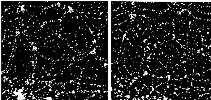
Рис. 12. Завершающие фазы эволюции группирования при моделировании нелинейного разрастания крупномасштабной структуры Вселенной (по Coles P. et Lung-Yih Shang в работе 251 )
