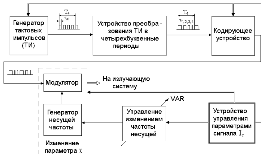
Рис. 11. Блок-схема формирования сигнала I_c
