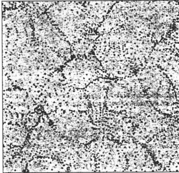
Рис. 13. Иллюстрация к возникновению плотных блиноподобных утолщений газа в ранней Вселенной; «блины» видны с ребра в виде линий, вдоль которых концентрируются частицы (по И.Д. Новикову 253 в работе 251 )
