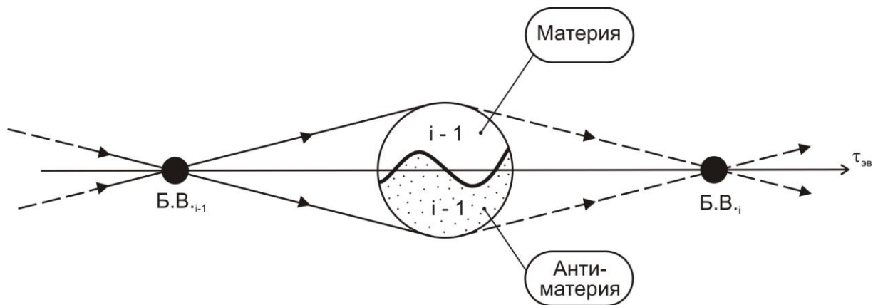
Рис. 16. Иллюстрация к лемме 16 в концепции циклических (пульсирующих) вселенных: в результате Большого взрыва B.V_{i-1} образуется (i-1) -я вселенная, например, наша Вселенная, которая далее стягивается в сингулярность для B.V_i в результате аннигиляции материи и антиматерии
