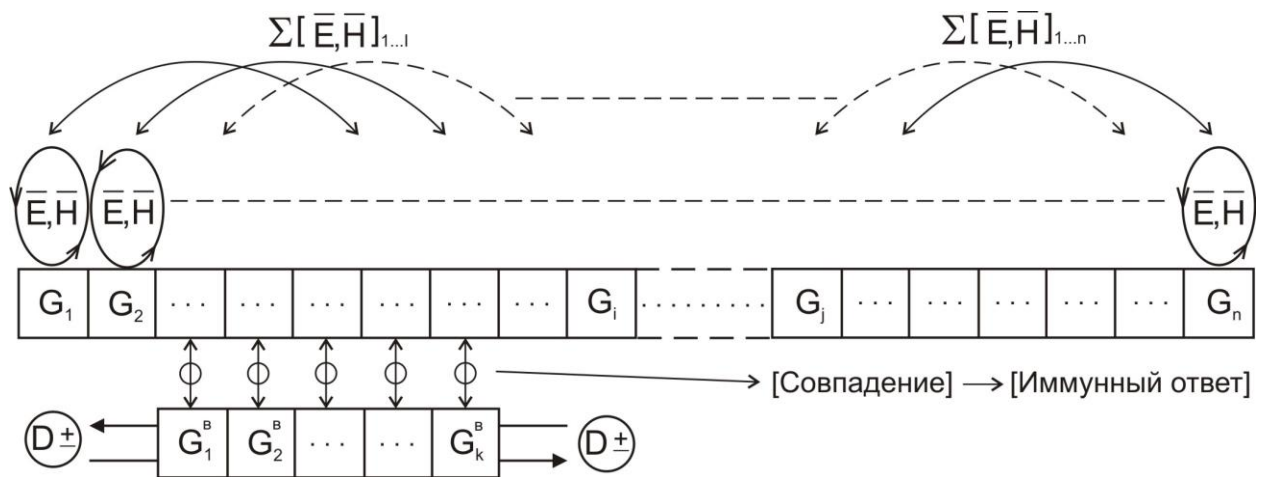
Рис. 21. Вещественно-полевая структура ДНК с геномом, содержащим последовательный набор генов G_1 G_2 \dots G_i \dots G_j \dots G_n ; \bar{E}, \bar{H} – зацикленные ЭМП i -го гена; \Sigma[\bar{E}, \bar{H}]_{1\dots n} – ЭМП, связывающие гены G_1 \dots G_n – каждую их пару в переборе 1\dots n , и гены G_1 \dots G_n в иерархии их кластеров; G_1^B, G_2^B \dots G_k^B – набор генов, в последовательности составляющих геном вируса; (D^\pm) – возвратно-поступательное «движение» ДНК(РНК) вируса вдоль ДНК многоклеточного организма (человека)
