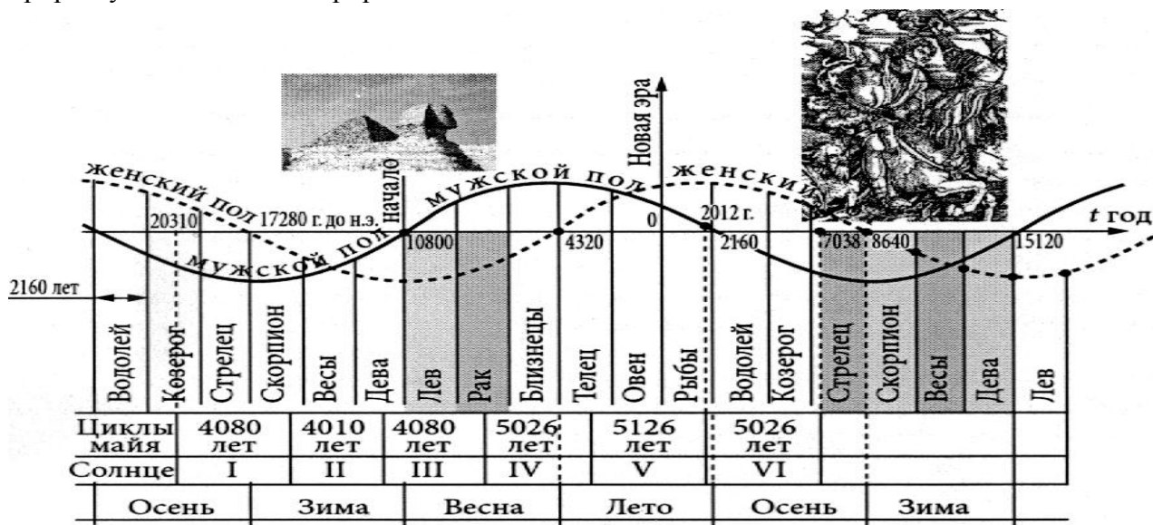
Рис. 2. График современного зодиакального года (10 800 до н.э. – 15 120 н.э.)
