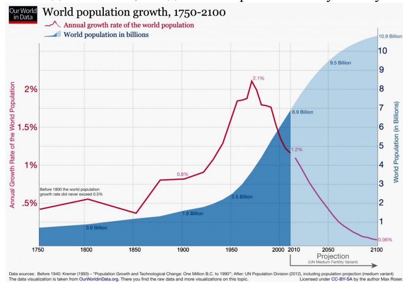
Рис. 1. График роста численности населения Земли с 1750 года по 2100 год. Сверху показан график прироста численности. Максимум прироста численности приходится на 1962 год. (ИНТЕРНЕТ ресурсы).
